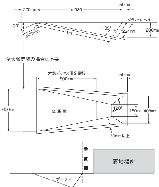
棒高跳用ボックス規格
