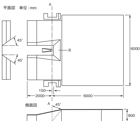
棒高跳用マット
